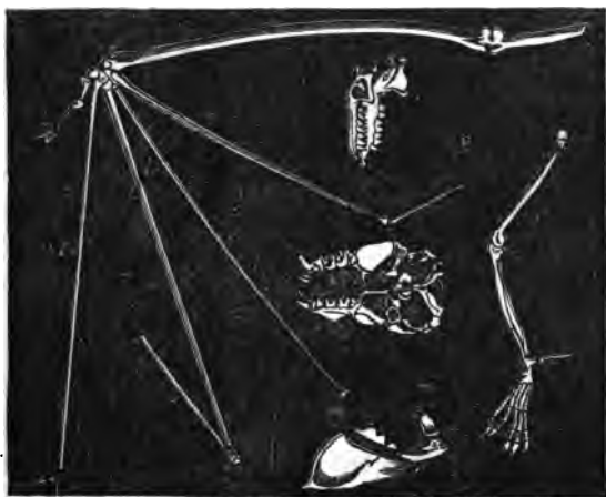
VESPERTILIO PARIISIENSIS. A Bat of the Eocene.
